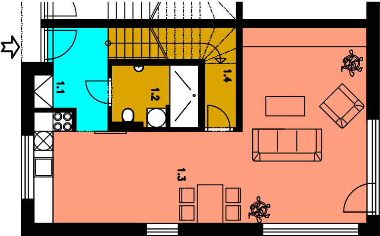
PŮDORYS PŘÍZEMÍ
