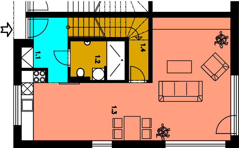
PŮDORYS PŘÍZEMÍ
